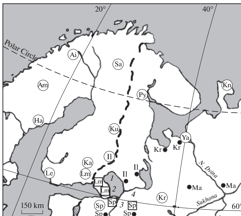
Рис. 1. Распространение кариотипических вариантов обыкновенной бурозубки Sorex araneus на Севере-Западе России и прилегающих территориях. Буквами в кружках обозначены места первоописания соответствующих рас в России (Kr – Kirillov, Kn – Kanin, Ku – Kuhmo, Py – Poyakonda, Sp – St. Petersburg, Ya – Yagry), в Финляндии (II – Ilomantsi, Ka – Kalvitsa, Le – Lemland, Lm – Lemi, Sa – Savukoski) и Швеции (Ai – Abisko, Am – Ammarnas, Ha – Hattsjo). Все известные по литературным данным локалитеты с кариотипированными S. araneus на данном участке в пределах России обозначены черными кружками, наши новые данные – буквами в квадратах (локалитеты 1–4). Пунктирная линия – граница России.
